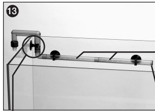
Abrazadera de ventosa
