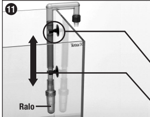
a) Exemplo de utilização Mola comprida
