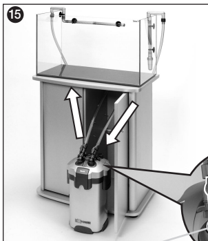
OUT = Auslass
