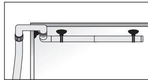
b) Beispiel: Kurze Clips
