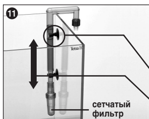
а) Пример использования Присоска с длинным зажимом
